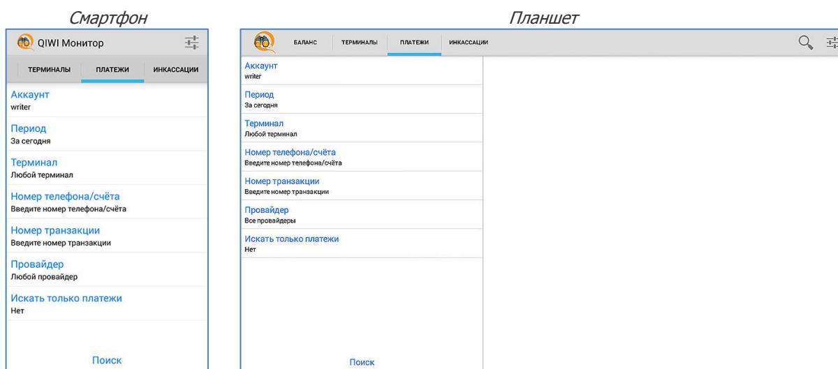
Рис. 10. Вкладка «Платежи»
