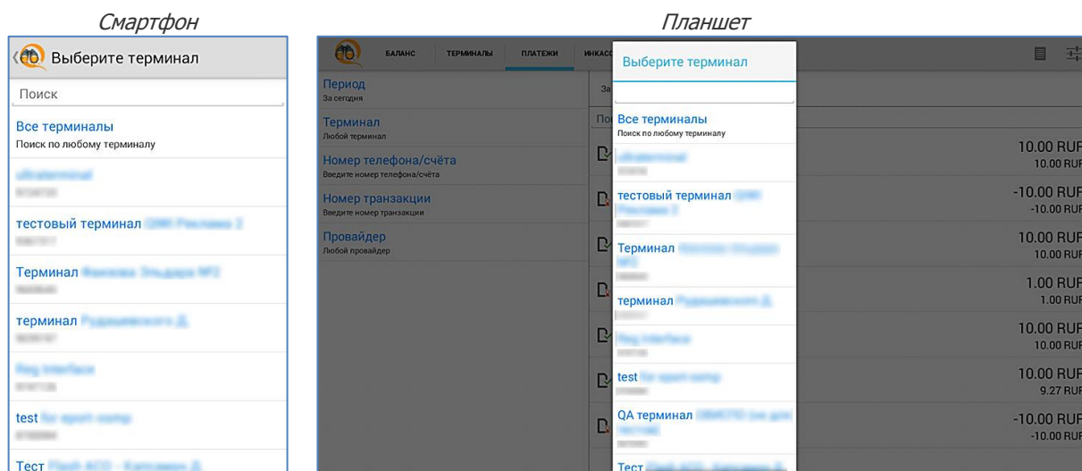
Рис. 13. Выбор терминала
