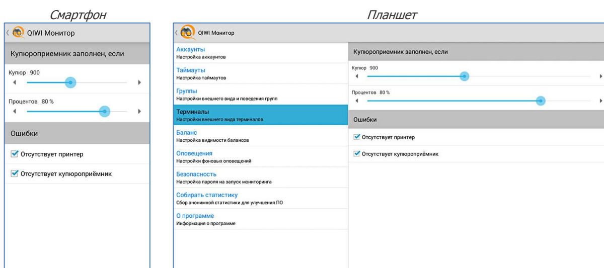
Рис. 28. Настройка терминалов
