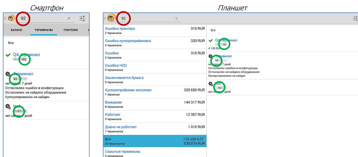
Рис. 5. Поиск терминала
