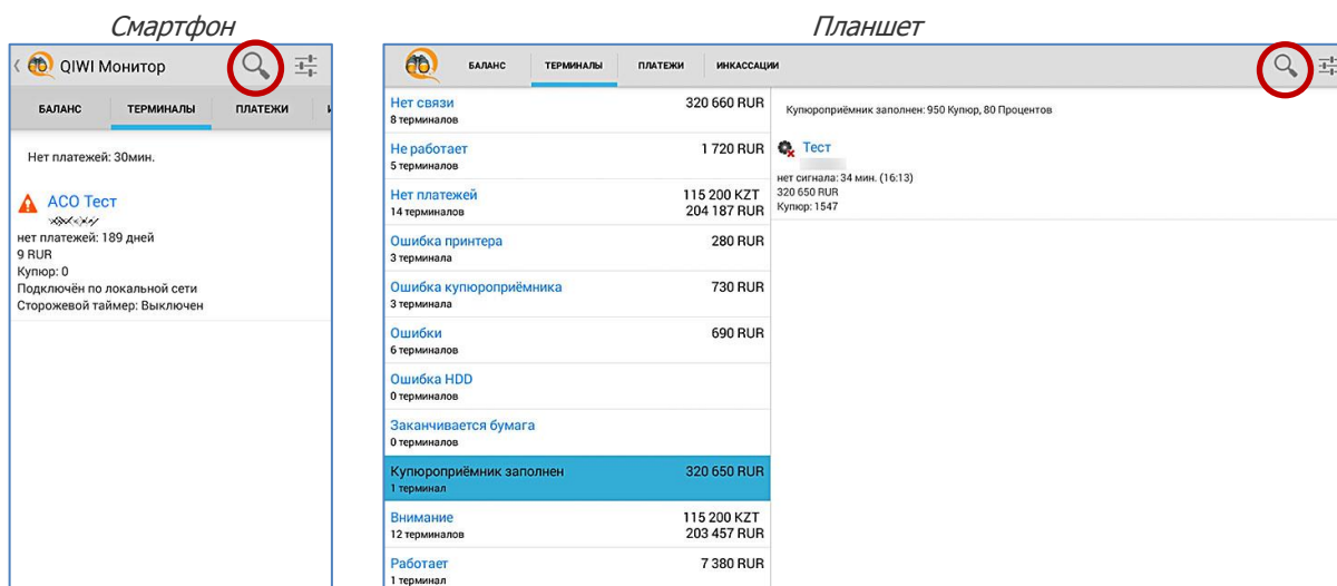
Рис. 4. Список терминалов
