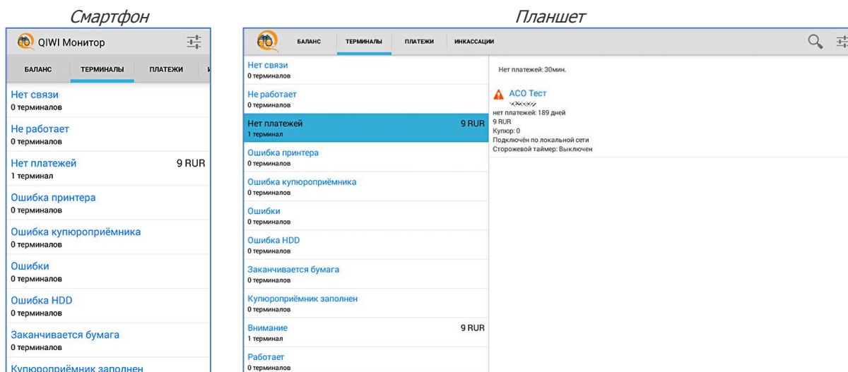
Рис. 3. Вкладка «Терминалы»
