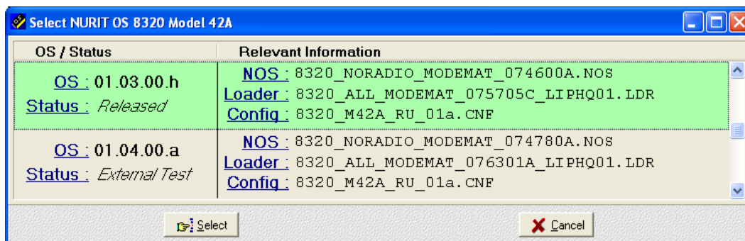
Рис. 6. Выбор прошивки
