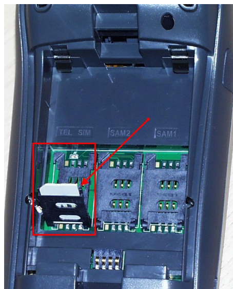
POS-терминал S-90
