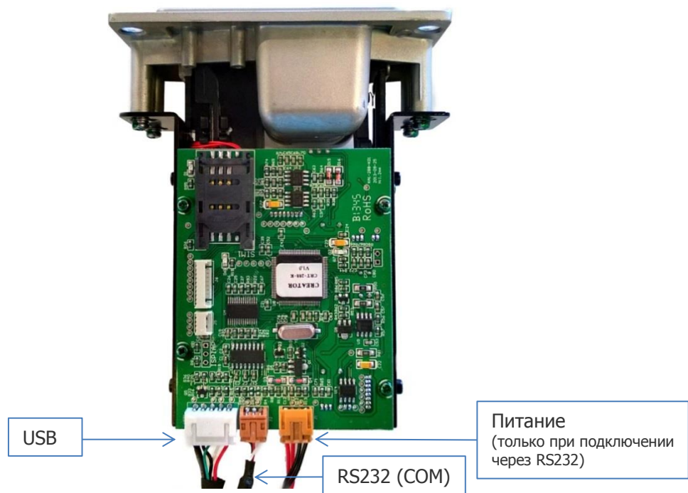
Рис. 1. Подключение устройства чтения карт CRT-288-K001
